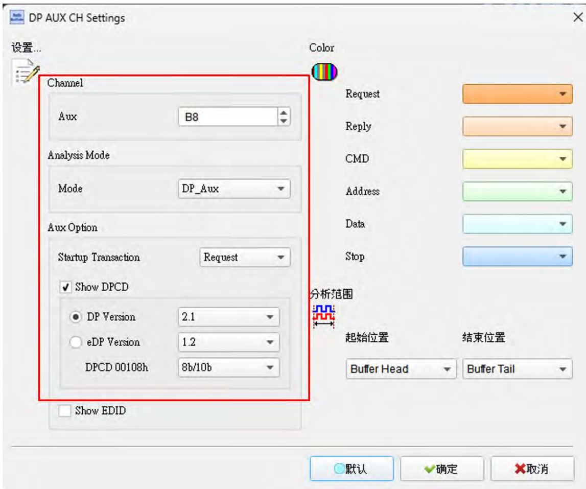
(3) 将 Sample Rate 采样率改为 20MHz 并将通道项目设置为 A0-B31 后即可开始抓取 DP_AUX
